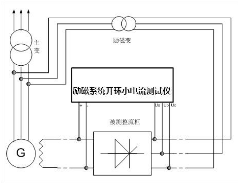
图 1 励磁系统开环小电流测试仪测试原理图
