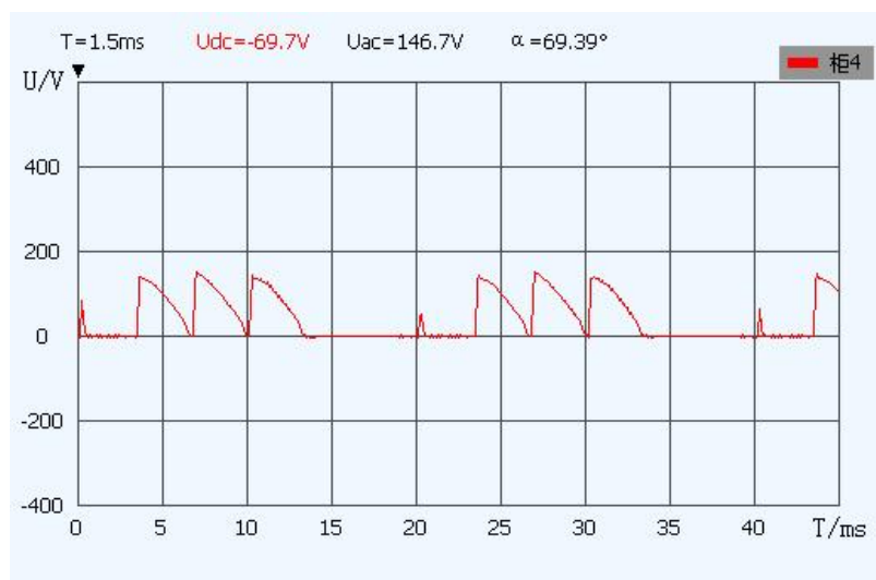
图 11 A+B-脉冲断线
