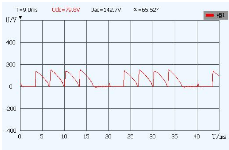
图8 A+脉冲断线
