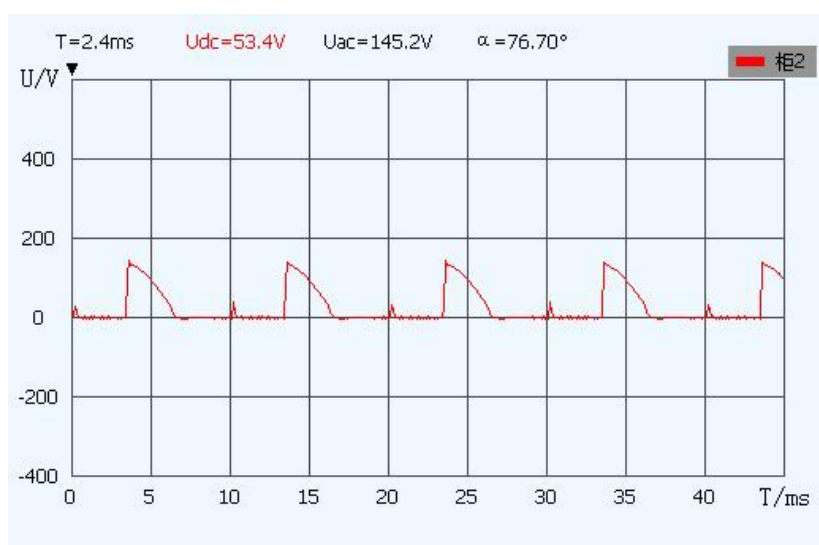
图 9 A+A- 脉冲断线
