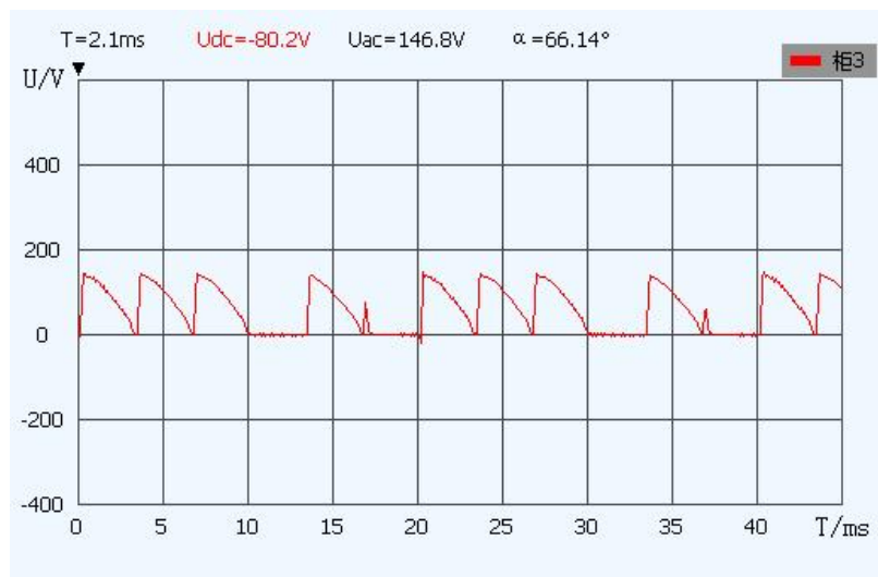
图 17 A+B-脉冲接反
