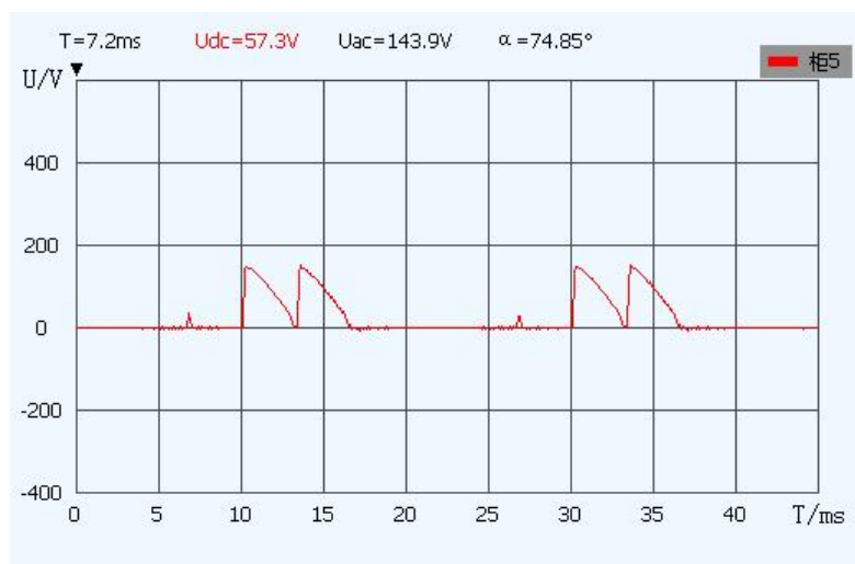
图 12 A+B+C-脉冲断线
