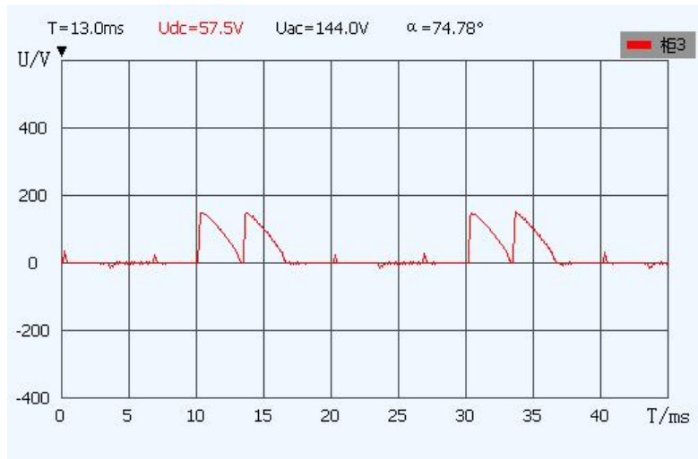
图 10 A+B+脉冲断线
