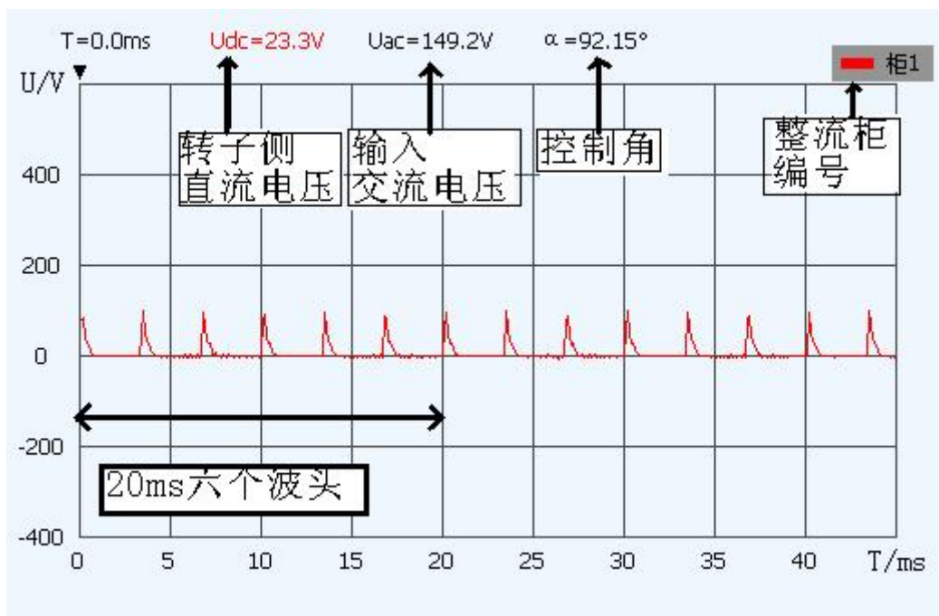
励磁系统开环小电流试验典型波形图
