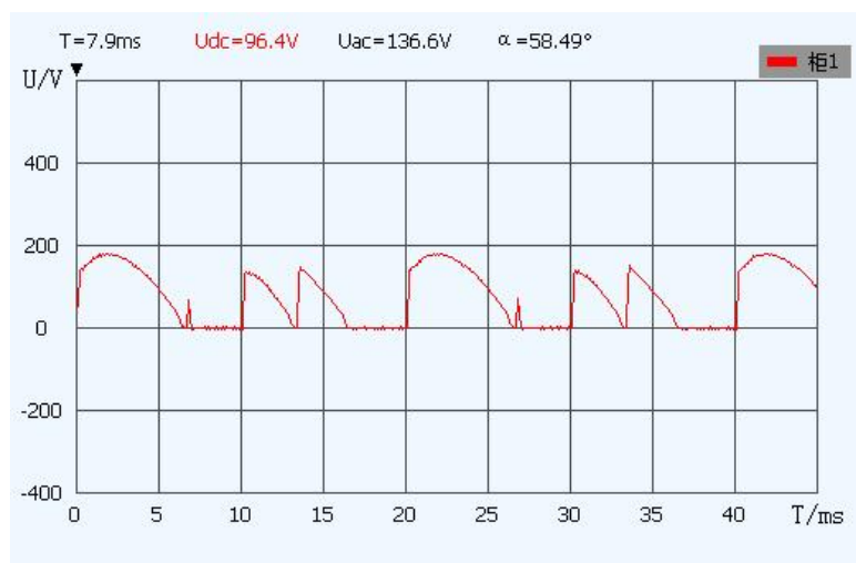
图 15 A+B+脉冲接反
