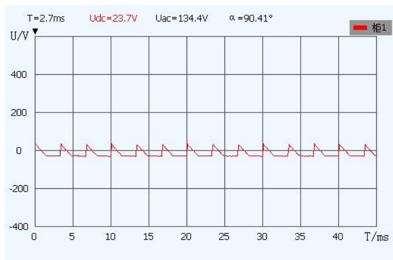
图 18 励磁系统开环小电流试验录波图
