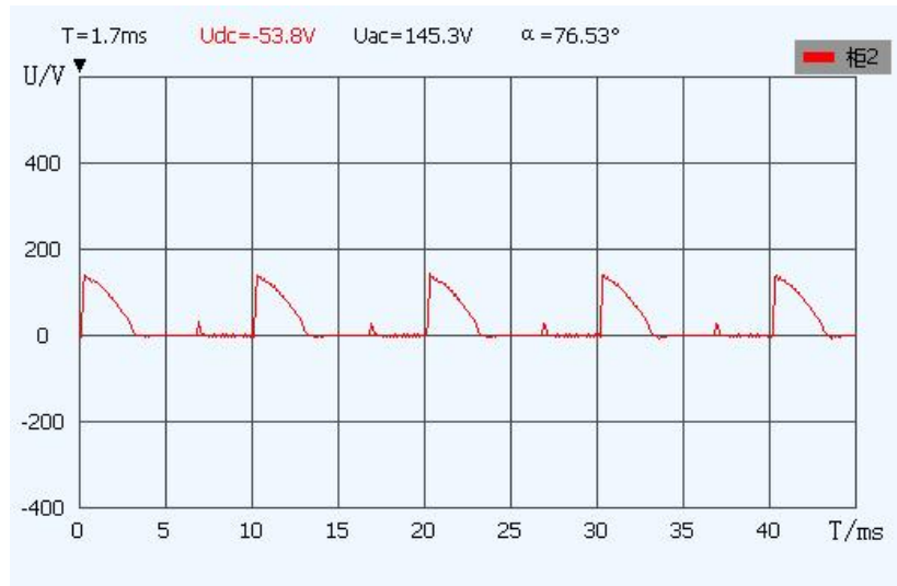
图 16 A+A-脉冲接反
