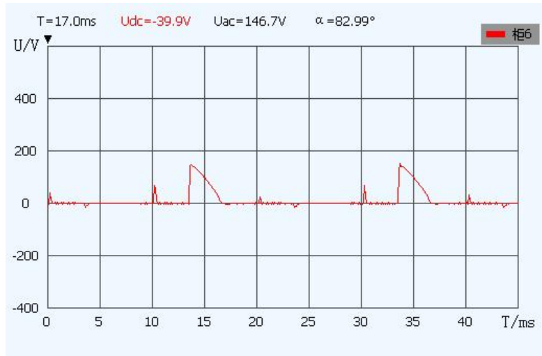
图 13 A+B+A-脉冲断线
